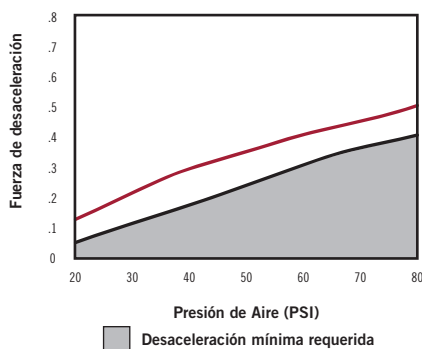
Desaceleración a 50 MPH
