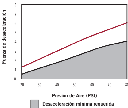
Desaceleración a 50 MPH
