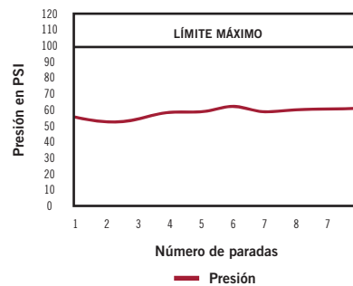
Potencia de frenado
